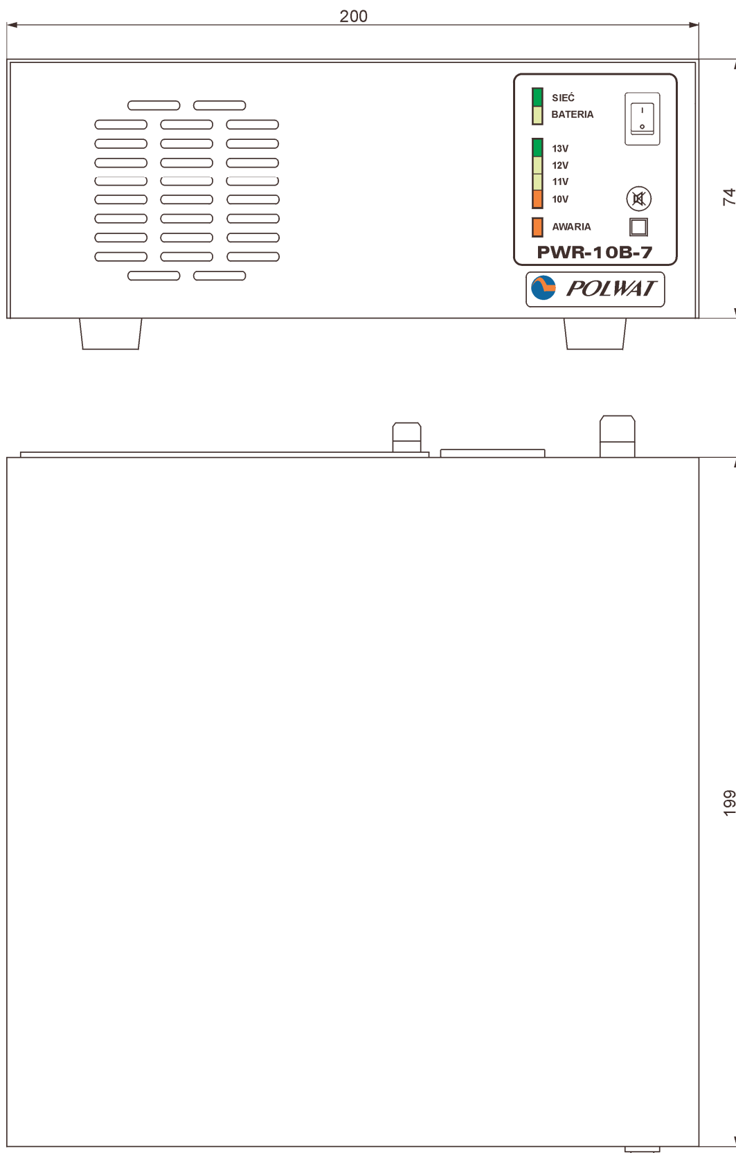
Rys.1. Wymiary gabarytowe zasilacza PWR-10B-7
